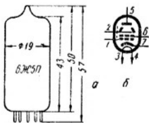
Рис. 233. Лампа 6Ж5П:
