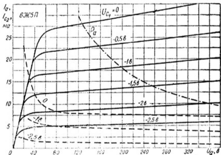
Рис. 234. Усредненные характеристики зависимости тока анода и тока второй сетки от напряжения на аноде при напряжении на второй сетке 150 в: — ток в цепи анода; — — ток в цепи второй сетки; - - - - наибольшая мощность, рассеиваемая на аноде.
