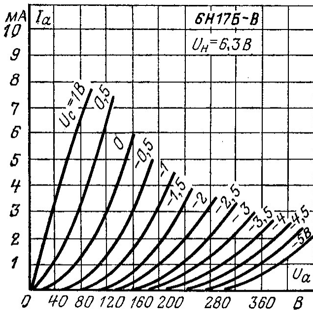
Анодные характеристики.
