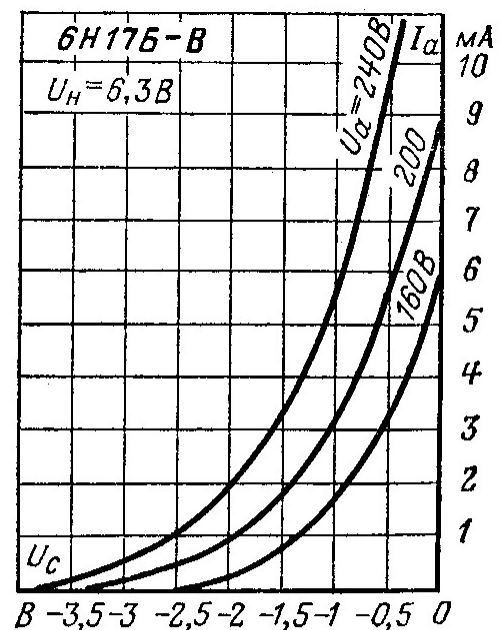
Анодно-сеточные характеристики.
