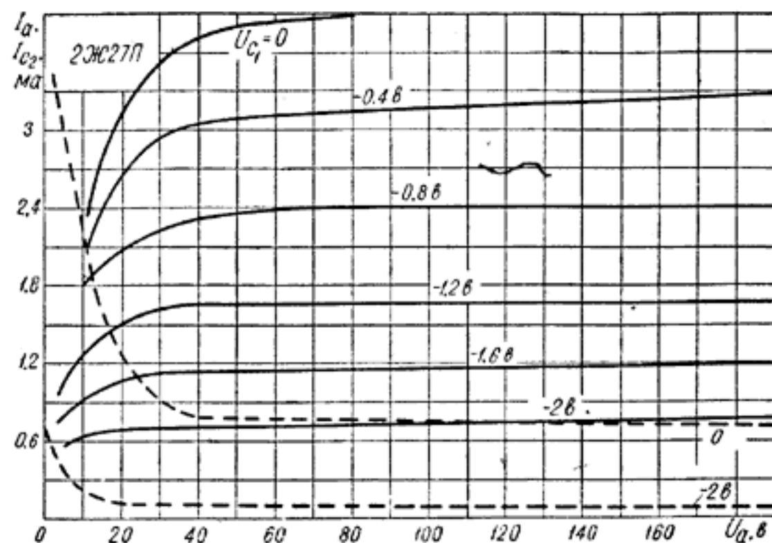
Рис. 97. Усредненные характеристики зависимости тока анода и тока второй сетки от напряжения на аноде при напряжении на второй сетке 45 в и напряжении на третьей сетке 0:
