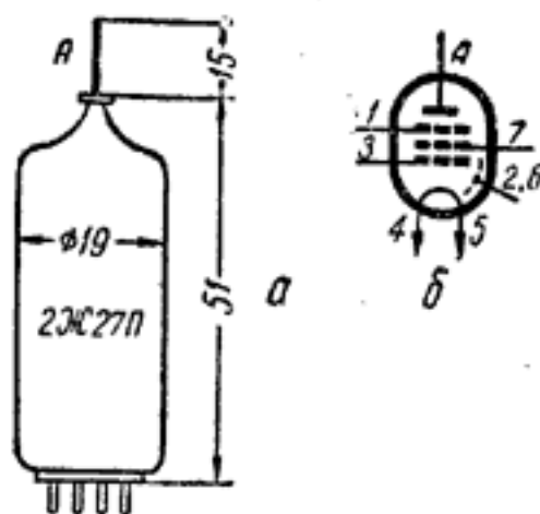
Рис. 96. Лампа 2Ж27П:
